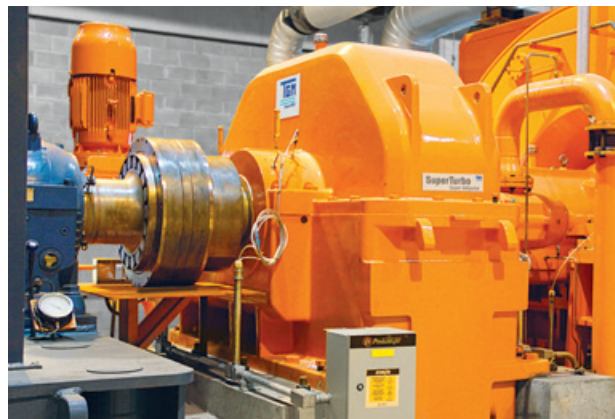
CERRADINHO - Chapadão do Céu, GO / Turbogenerador - 45 MW SuperTurbo - ST 710
